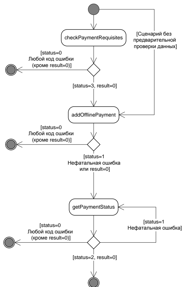
Рис. 6. Сценарий оффлайн проведения платежа
